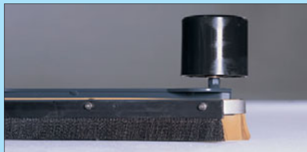
Der Saugfuß ist zusätzlich mit einem Besenleiste für die Aufnahme von Grobschmutz ausgestattet.
